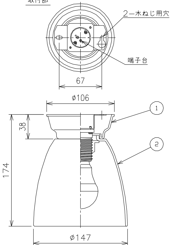
取付部
